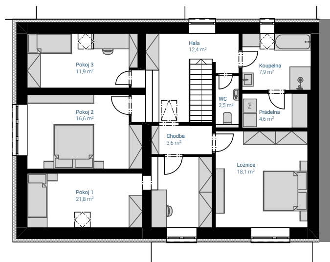
Půdorys podkroví
