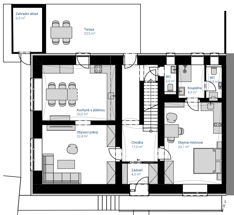
Půdorys 1. podlaží
