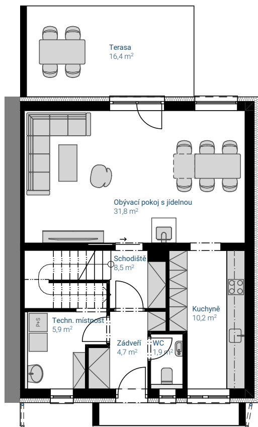
Půdorys 1. podlaží
